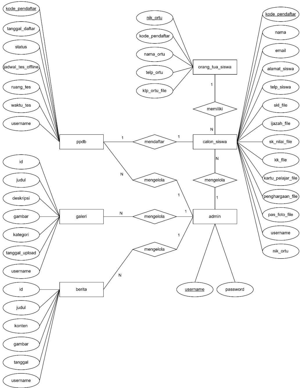
Gambar 4. ERD Sistem PPDB
