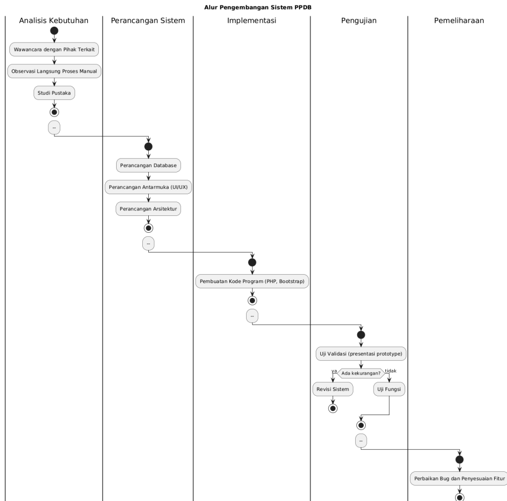
Gambar 1. Alur Pengembangan Model Waterfall
